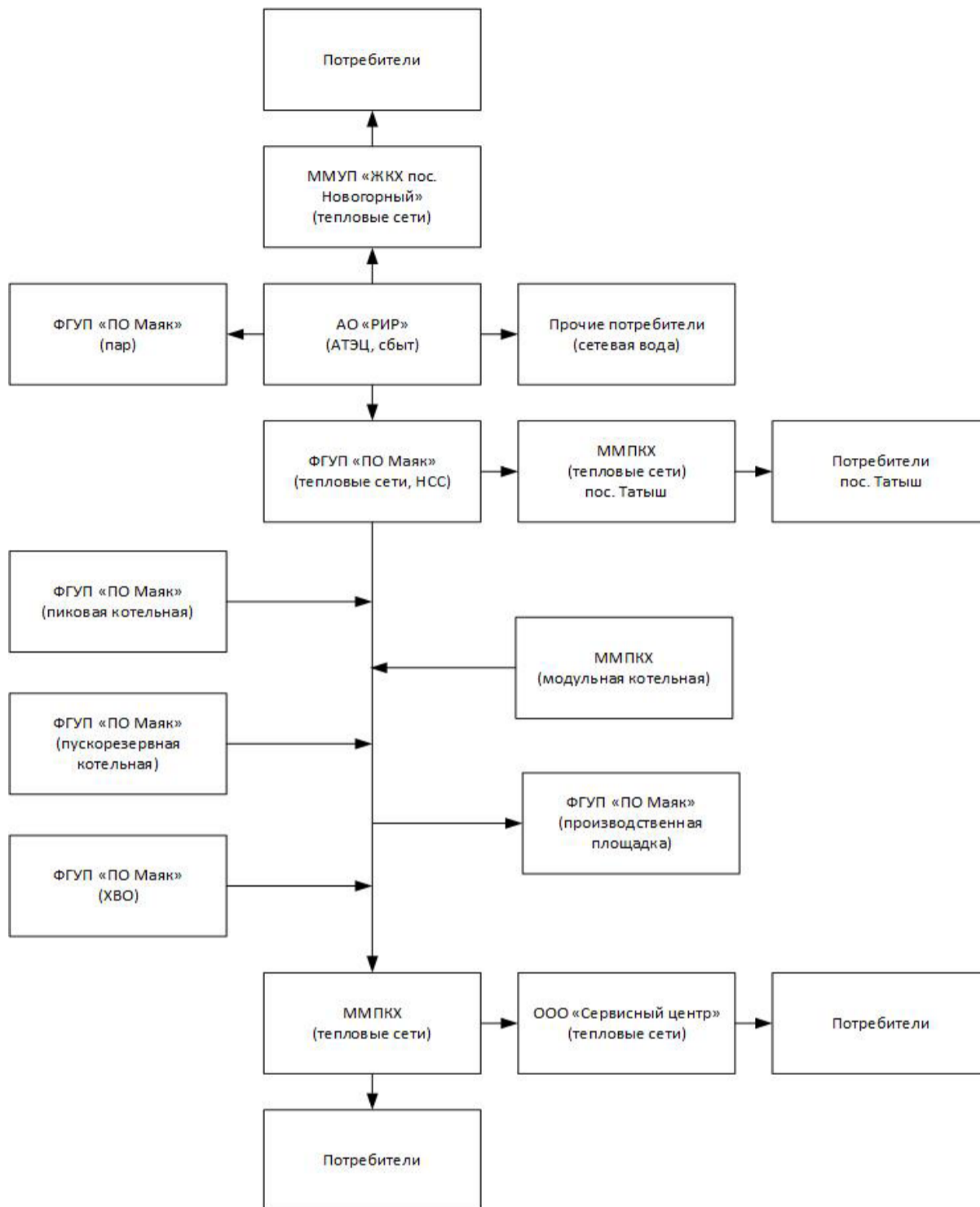
Рисунок 1-1 - Структурная схема зон эксплуатационной ответственности теплоснабжающих организаций в системе «АТЭЦ+Пиковая котельная»
